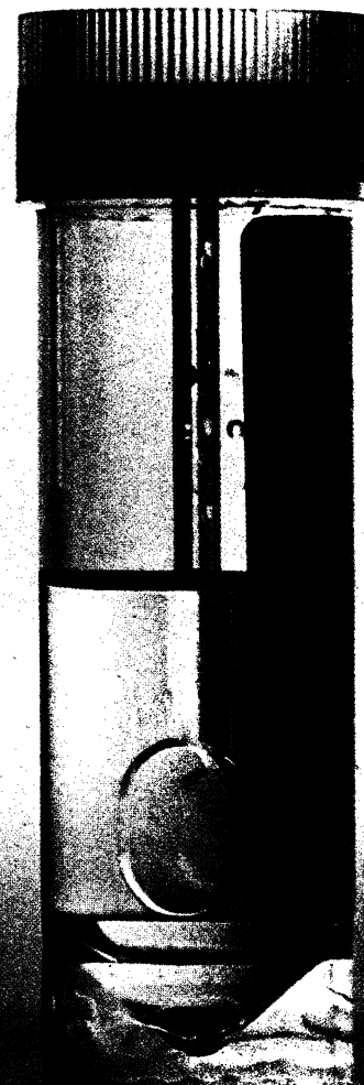
Klebsiella pneumoniae
